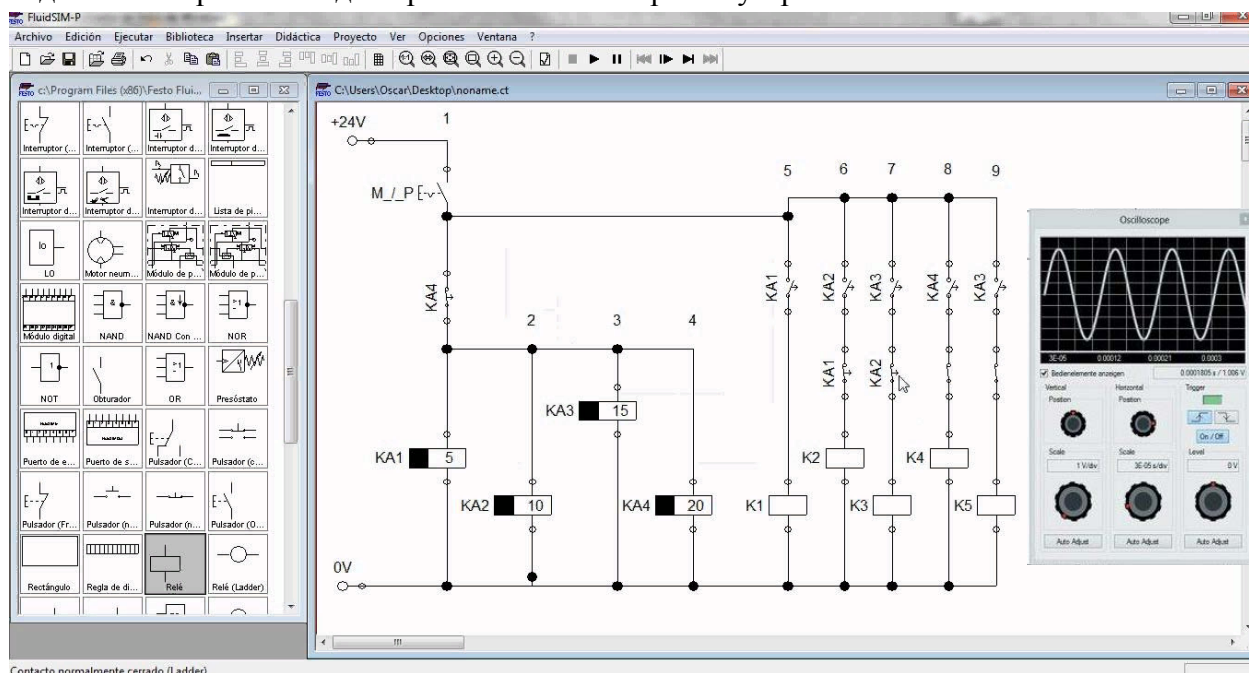
Рисунок 2 – Моделирование электрической цепи
